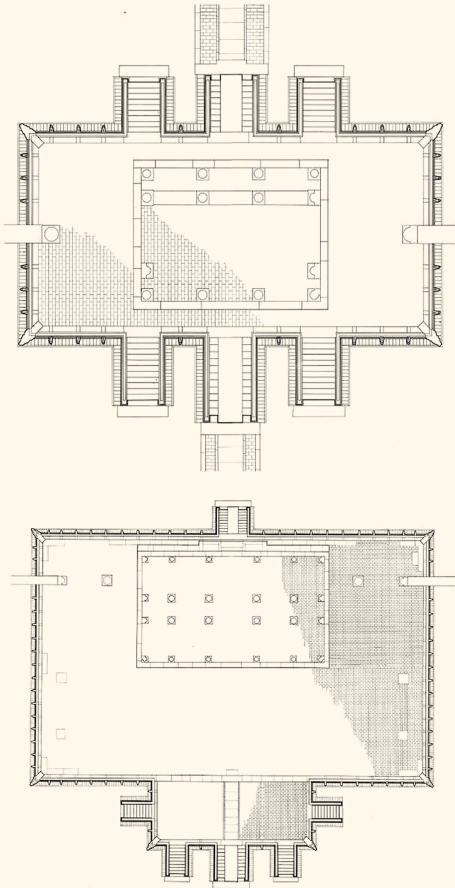
明永陵祿恩門、祿恩殿现状测绘图 天津大学建筑学院绘制
