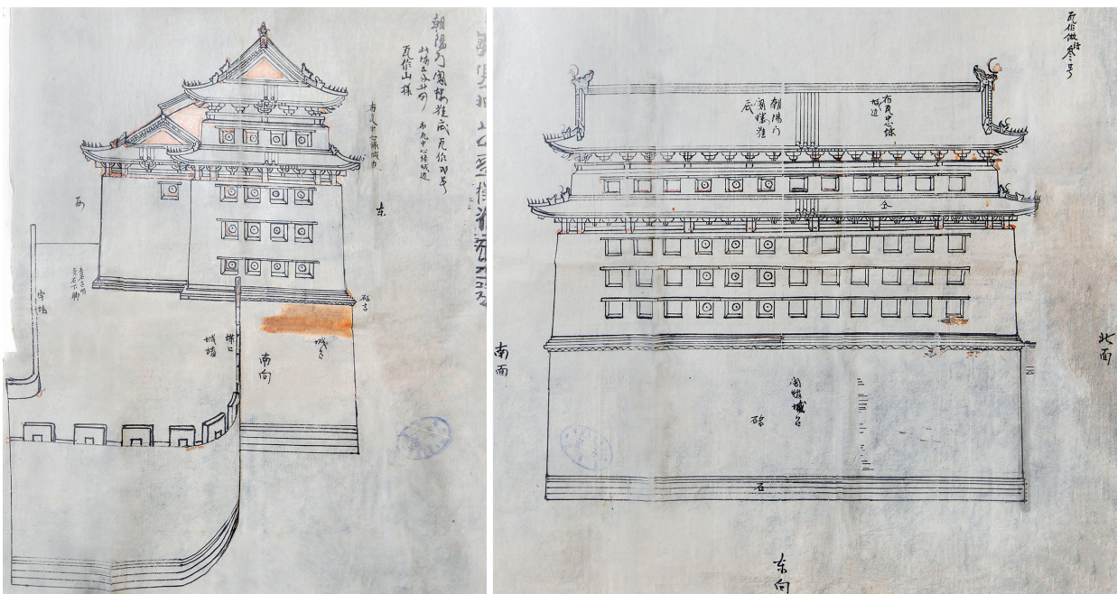
〔图十〕人39朝阳门箭楼南立样(左)东立样(右)
