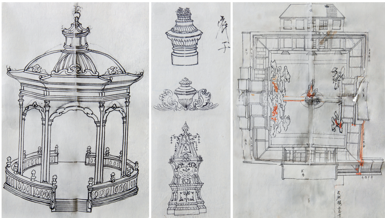
〔图六〕人43中海海晏堂或集灵囿洋式井亭立样(左)、人26中海海晏堂洋式鼎炉立样(中)、人48中海后照楼地盘并立样(右)
