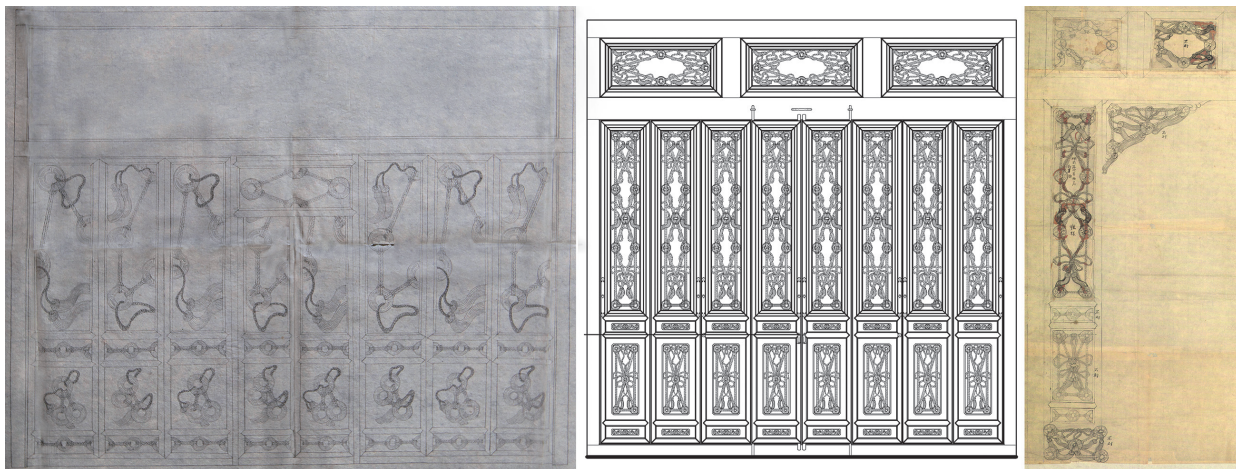
[图十二] 人32五抹榻扇八扇立样(左)、颐和园谐趣园涵远堂西次间后檐西缝西立面图(中)、 图354-1773颐和园谐趣园涵远堂内檐装修落地罩、天然罩立样(局部)(右) 天津大学建筑学院测绘
