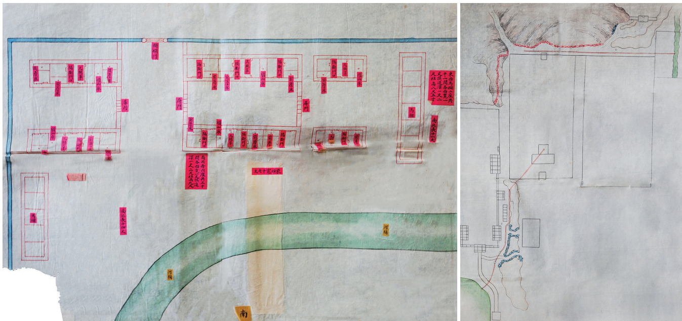
〔图二〕人1颐和园东宫门外迤南马厂墙内添修外边各项值房地盘样(左)、人21颐和园德和园大戏楼引水地盘样(右)
