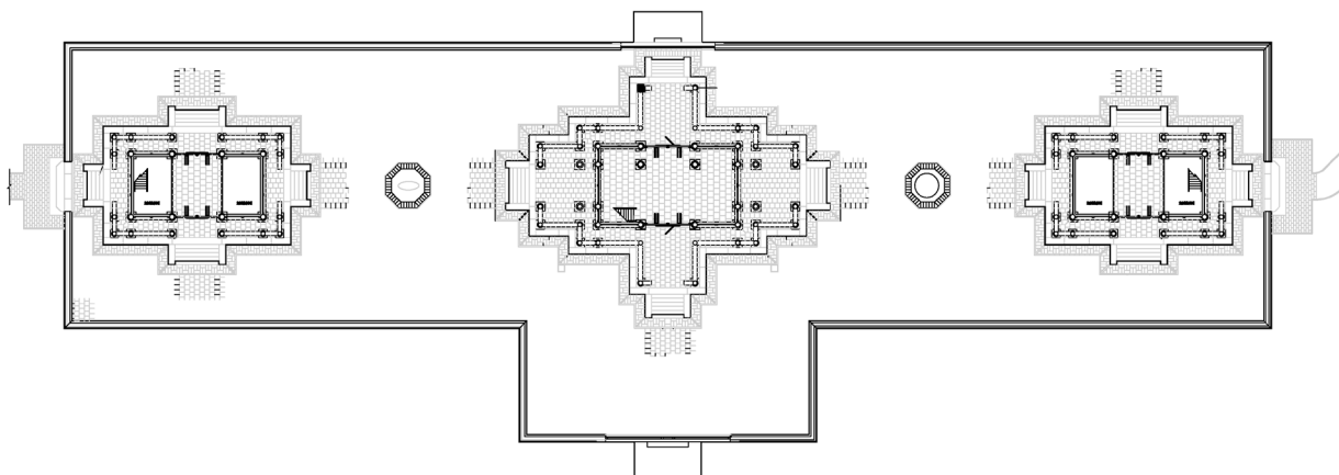
〔图四〕景明楼及其配楼平面图 天津大学建筑学院测绘
