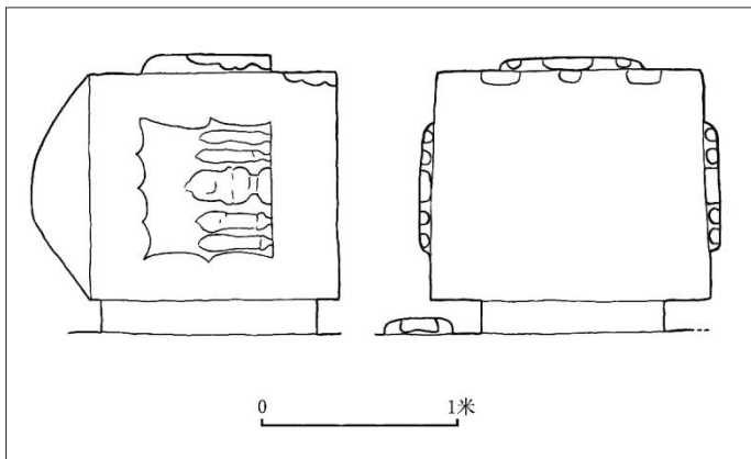
〔图七十九〕净居寺新1窟平面图
