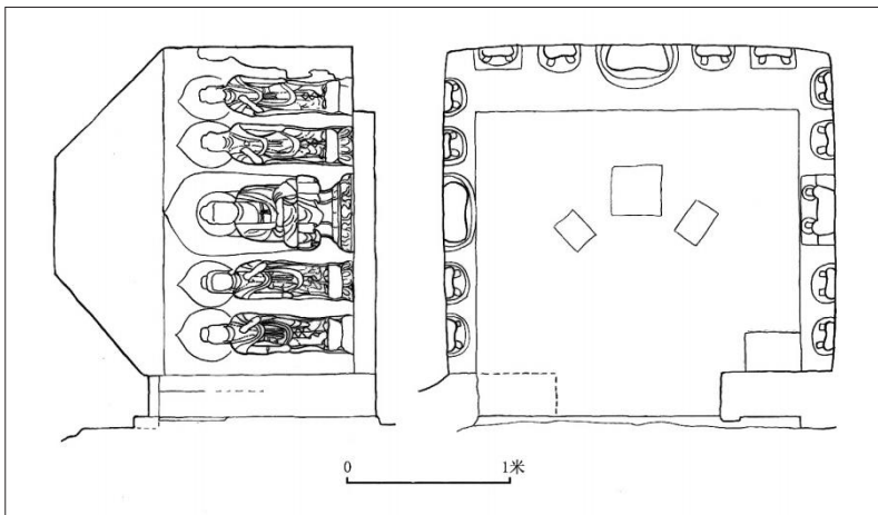
〔图十六〕净居寺第2窟平面图
