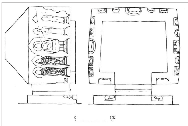
〔图四十二〕净居寺第4窟平面剖视图
