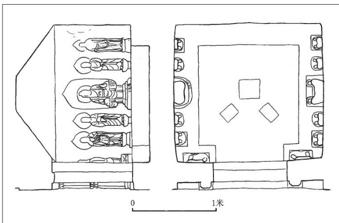
〔图三十〕净居寺第3窟平面图
