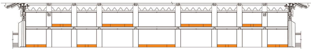
图 5-3 乾清宫纵剖面图
