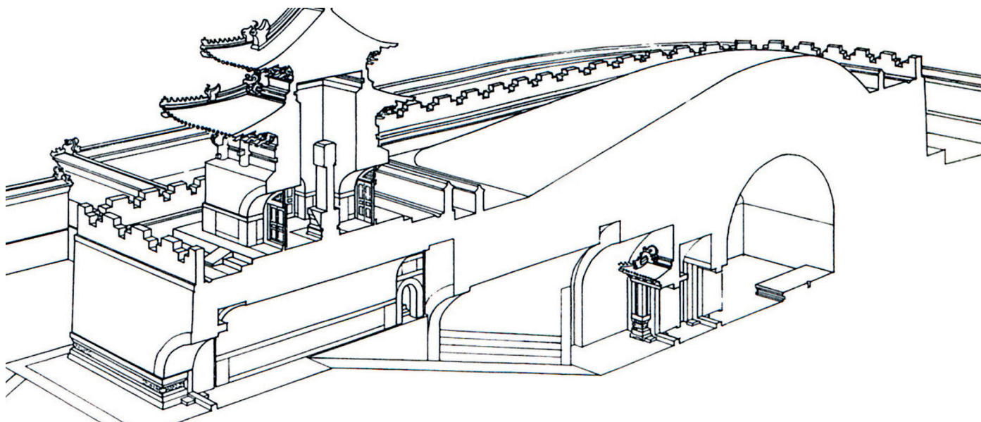
慈禧陵地宫剖面图
