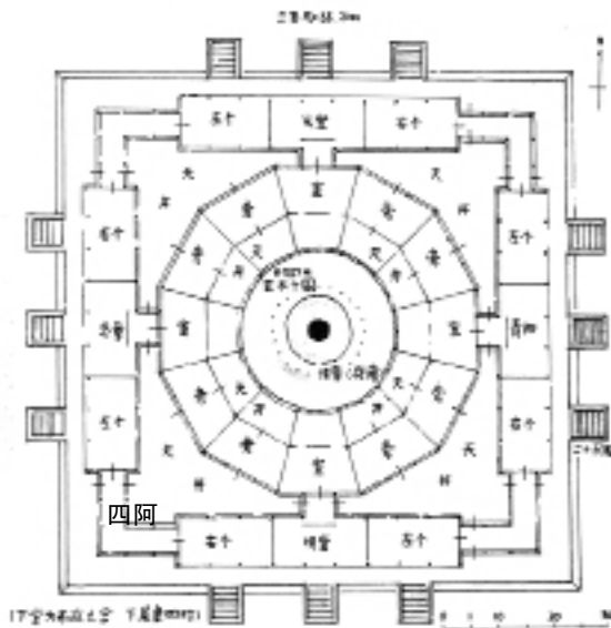
图5 河南洛阳武则天明堂遗址复原平面图
