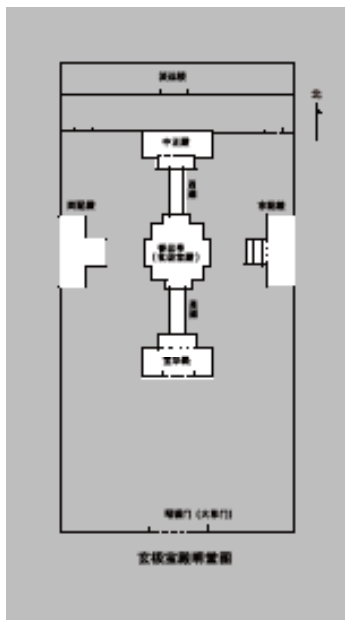
图7 中正殿区“十”字形平面图
