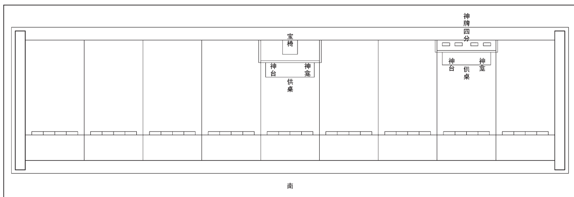
〔图十六〕瑞应宫晏安殿平面图 摹自样式雷图
