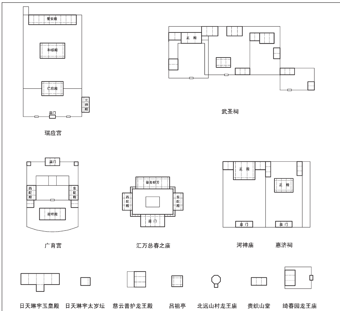
〔图十五〕圆明三园部分祀庙祠宇建筑平面示意图 作者自绘
