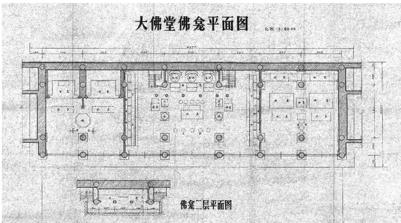
〔图七〕大佛堂平面图
