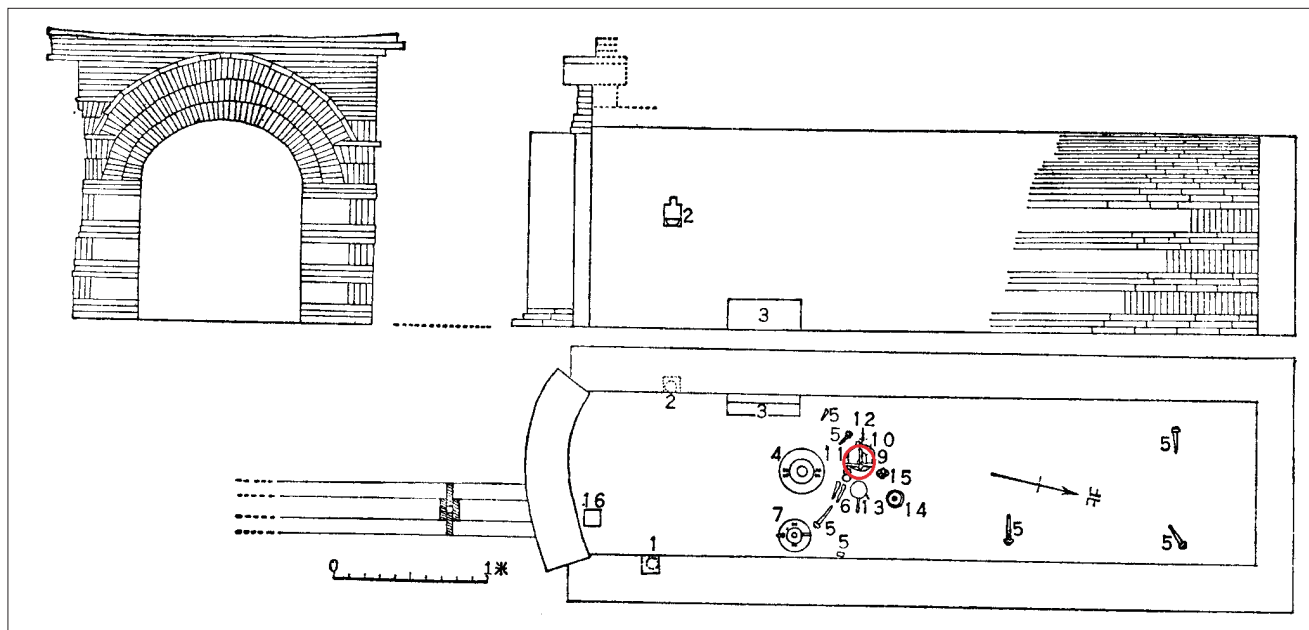
〔图三〕象山5号墓(王闰之墓)平面图
