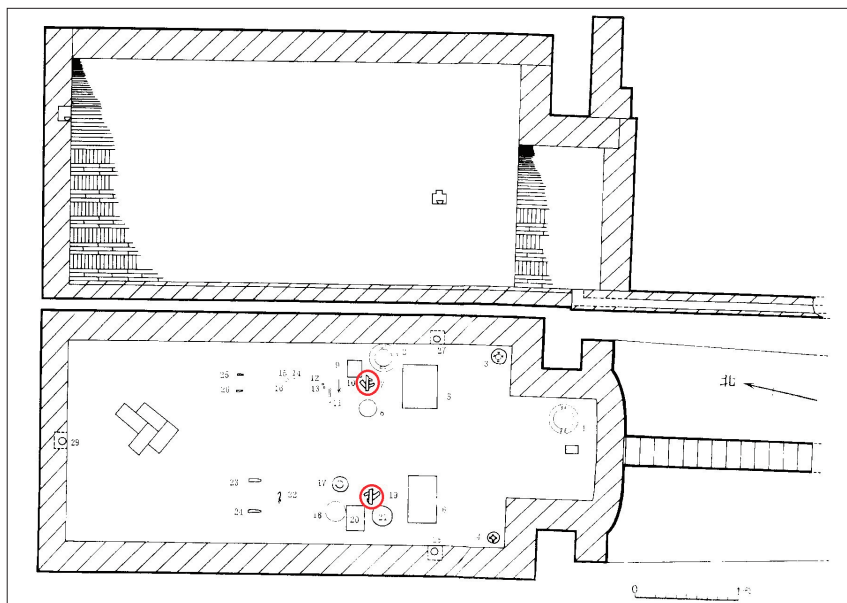
〔图五:1〕象山9号墓平面图
