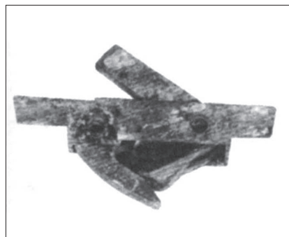
〔图五:3〕象山9号墓铜弩机 (M9:7)
